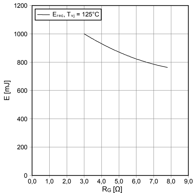
Schaltverluste Diode-Brems-Chopper (typisch) switching losses Diode-brake-chopper (typical) E_{rec} = f(R_G) I_F = 250 \text{ A}, V_{CE} = 3600 \text{ V}
