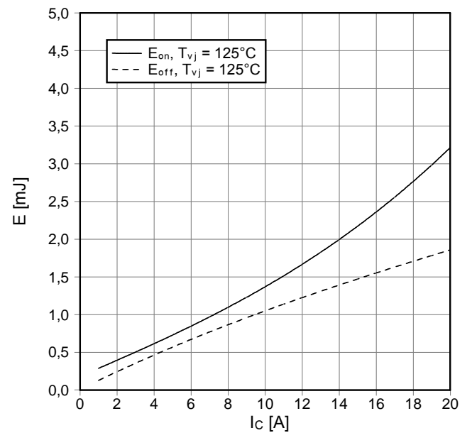
Schaltverluste IGBT-Wechselr. (typisch) switching losses IGBT-inverter (typical) E_{on} = f(I_c) , E_{off} = f(I_c) V_{GE} = \pm 15\text{ V} , R_{Gon} = 100\ \Omega , R_{Goff} = 100\ \Omega , V_{CE} = 600\text{ V}
