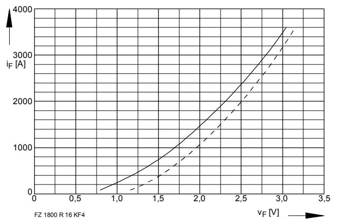
FZ 1800 R 16 KF4 Bild / Fig. 6 Durchlaßkennlinie der Inversdiode (typisch) Forward characteristic of the inverse diode (typical) ..... t_{vj} = 25^\circ C — t_{vj} = 125^\circ C
