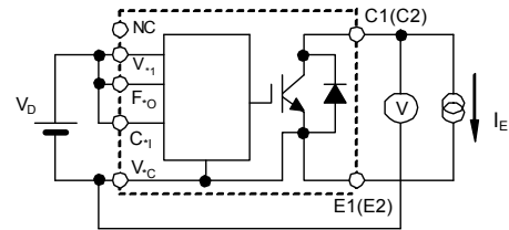
Fig. 2 V_{EC} Test
